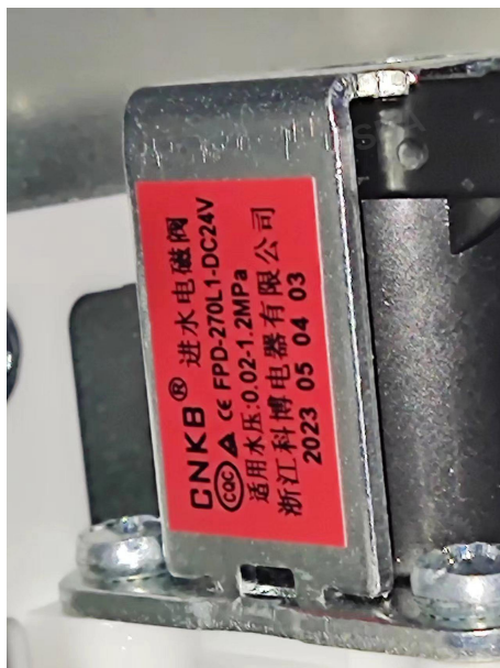
进水电磁阀
